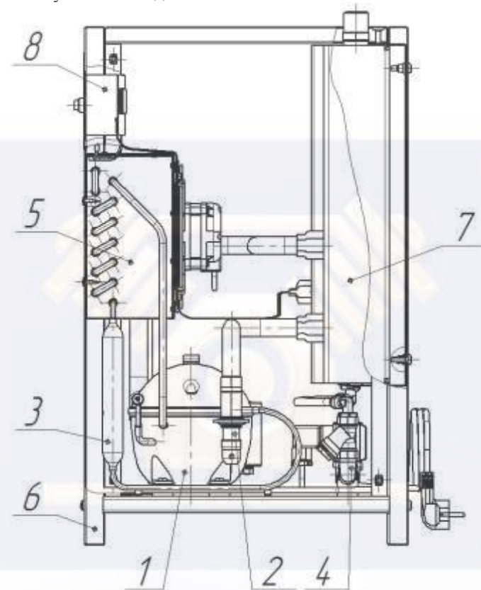
Рисунок 2 Основные узлы осушителя
