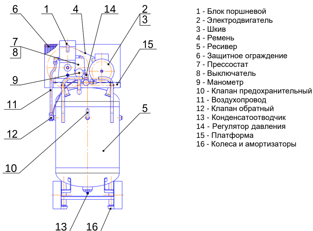
Рисунок 7 - Общий вид компрессоров СБ4/С-100.AB360AB, СБ4/С-100.AB360B
