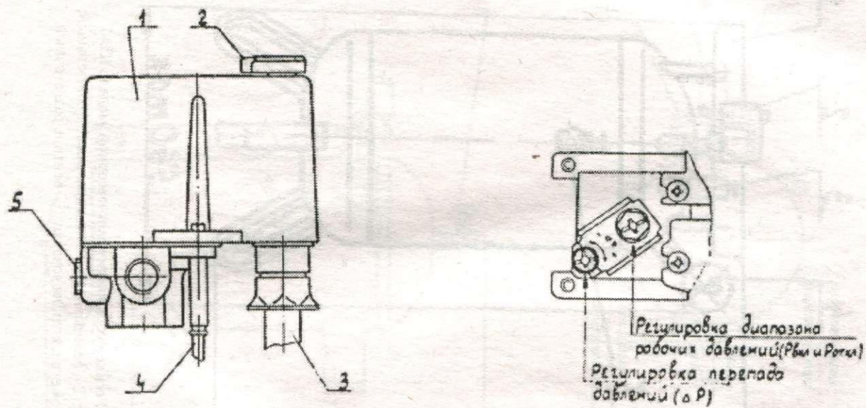
Рис. 7. Реле давления MDR 3/11 1 – кожух; 2 – переключатель; 3 – кабель; 4 – разгрузочная трубка; 5 – заглушка.
