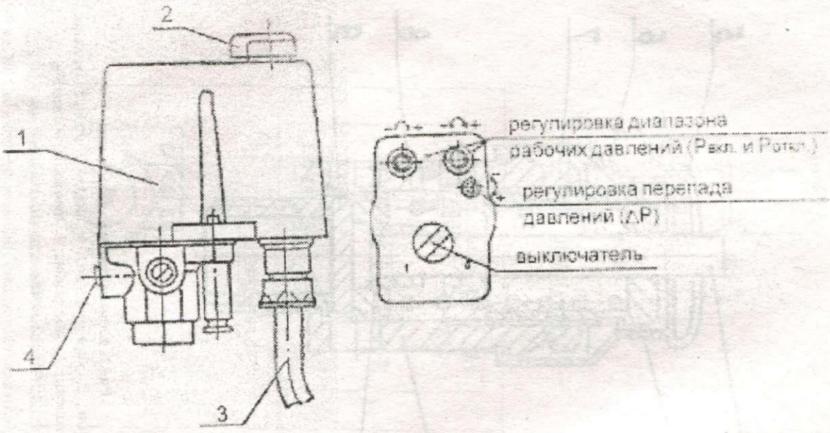
Рис. 7а. Реле давления MDR 2/11 1 – кожух; 2 – выключатель; 3 – кабель; 4 – заглушка.
