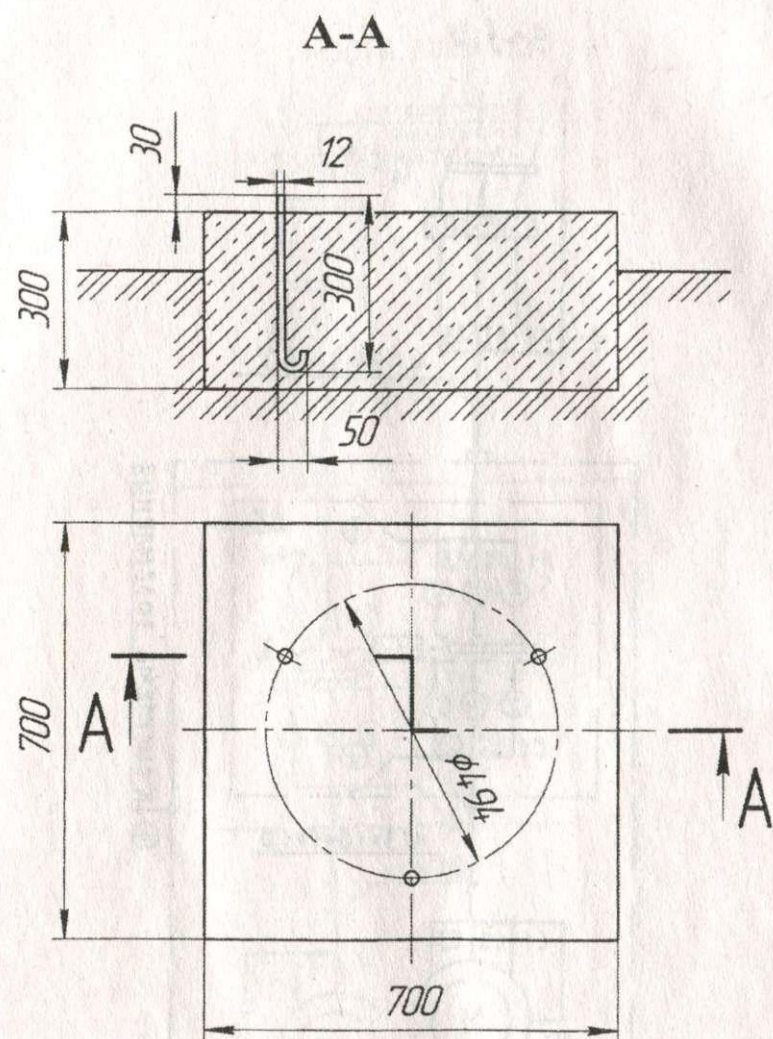
Рис. 13. План расположения фундаментных болтов установки КВ-7
