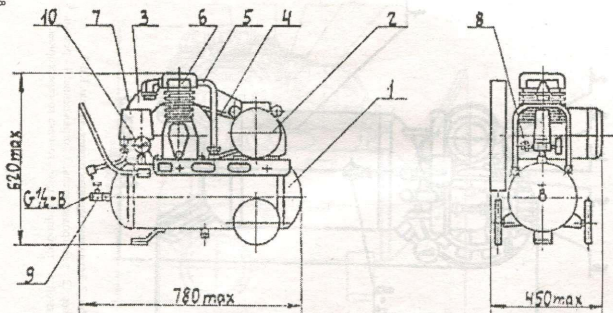
Рис. 3. Установка компрессорная, модель K-29, модель K29-01
