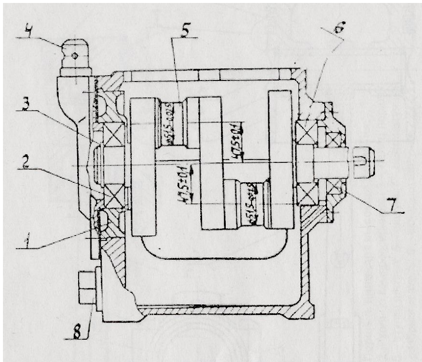
Рис. 5. Картер:
