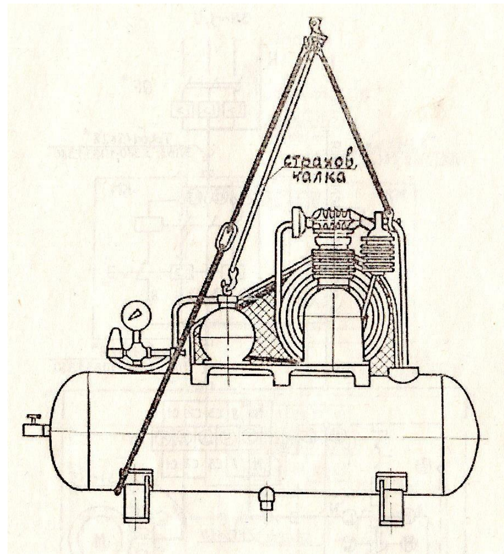
Рис. 19. Схема строповки компрессора модель C415M.
